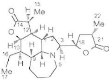
Neotuberostemonin
